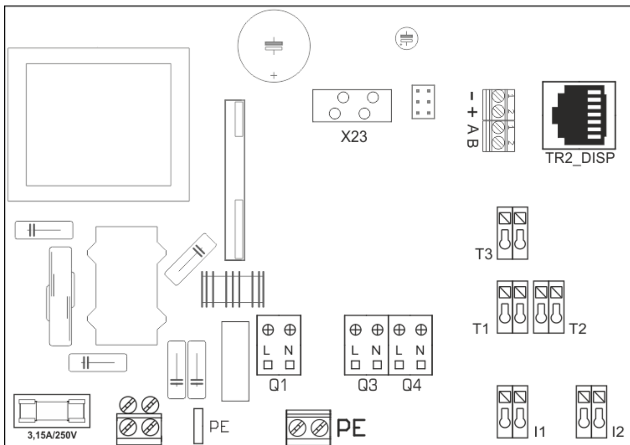
Питание 230 В
